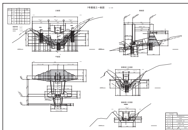
構造図
